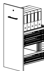
Telaio di serie capienza 6 dox + telaio porta cartelle + ripiano + 2 cassetti Standard frame capacity 6 dox + pull-out frame for hanging files + shelf + 2 drawers L 47,5 - P 82,5 - H 115
