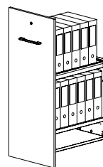
Telaio di serie capienza 12 dox + ripiano Standard frame capacity 12 dox + shelf L 47,5 - P 82,5 - H 115
