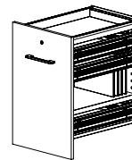
Telaio di serie + telaio porta cartelle + ripiano + 2 cassetti Standard frame + pull-out frame for hanging files + shelf + 2 drawers L 47,5 - P 82,5 - H 74
