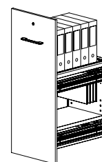
Telaio di serie capienza 6 dox + telaio porta cancelleria + ripiano + cassetto Standard frame capacity 6 dox + pull-out frame for hanging files + shelf + drawer L 47,5 - P 82,5 - H 115
