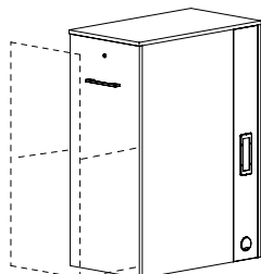
Mobile laterale per affianco a scrivania con telaio apribile a tutt'altezza Gruppo prese sul lato interno Side cabinet for desk with full height drawer Socket system on internal side L 47,5 - P 82,5 - H 115
