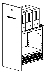
Telaio di serie capienza 12 dox con ripiano + cassetto Standard frame with shelf capacity 12 dox + drawer L 47,5 - P 82,5 - H 115
