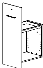
Telaio di serie Standard frame L 47,5 - P 82,5 - H 115
