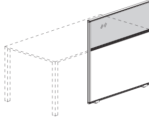
Parete divisoria da terra, parte inferiore cieca, in eco-legno o rivestita in tessuto, con parte superiore in doppio vetro trasparente Partition with eco friendly wood or fabric low part and trasparent double glass upper part L 160/180/200 - P 160 - H 74
