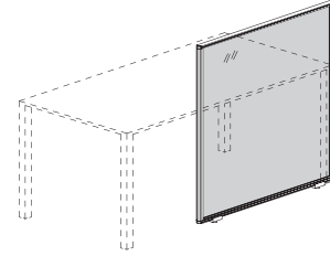
Parete divisoria con doppio vetro trasparente Partition with trasparent double glass L 60/70/80/90/100/120 - P 4 - H 115
