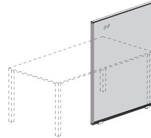
Parete divisoria con doppio vetro trasparente Trasparent double glass partition L 60/70/80/90/100/120 - P 4 - H 155
