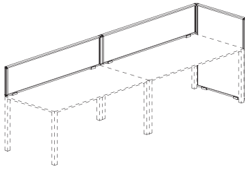
Composizione di schermi sopra-scrivania e parete divisoria laterale cieca in eco-legno o rivestite in tessuto Frontal screens and lateral eco friendly wood or fabric partition
