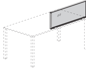
Schermo divisorio frontale con doppio vetro trasparente Double glass frontal screen L 60/80/100/120/140/160/180/200 - P 4 - H 40 (+74 cm)
